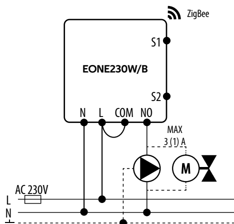
б) Схема подключения к насосу/сервоприводу
