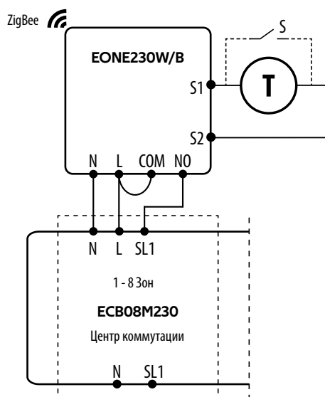
в) Схема подключения к центру коммутации
