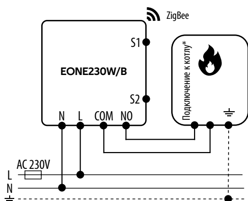
а) Схема подключения к газовому котлу
